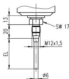
TP26 / TW39 ... T427 mit Gewinde M12x1,5 metallisch dichtend für Einschweißmuffe zem / TP26
