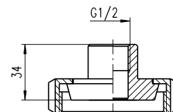
zfl / MG ... - TP16 Kegelstützen DIN 11851 DN25 ... DN50
