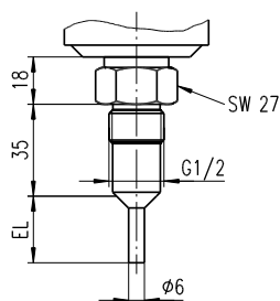
TP16 / TW39 ... T215 mit Gewinde G1/2 metallisch dichtend für Einschweißmuffe zem / TP16
