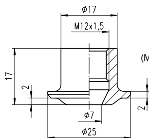
zem / TP26K Einschweißmuffe TP26 mit Kragen Art.-Nr. 07002001
